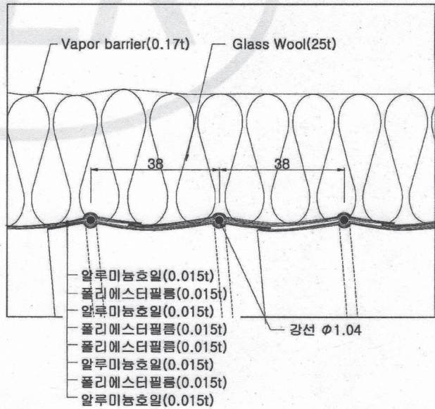
A부분 상세도
