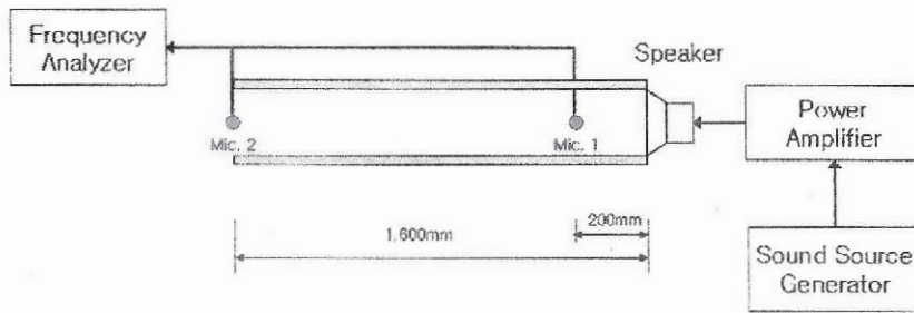
[그림 2] 측정방법
