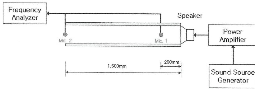
[그림 2] 측정방법
