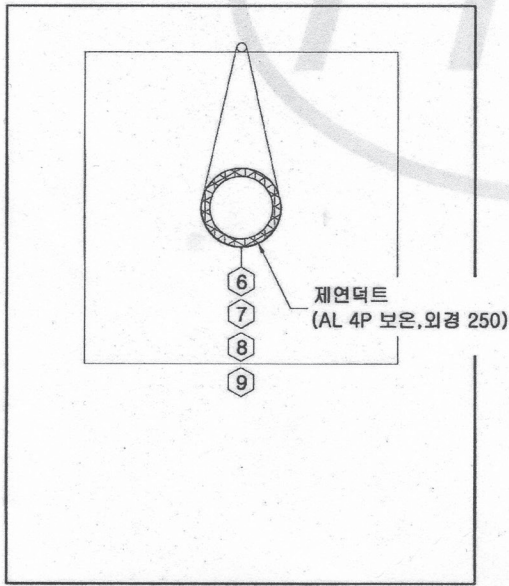
정면도
